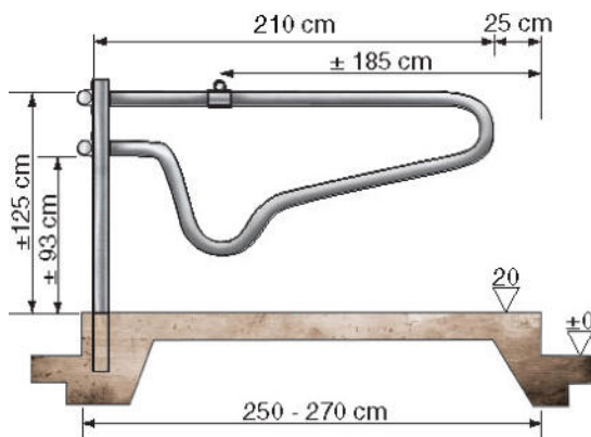
versch. Arten von Lieboxenabtrennungen Preis siehe Paturakatalog bis 12% Rabatt
